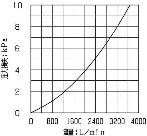
流量特性
