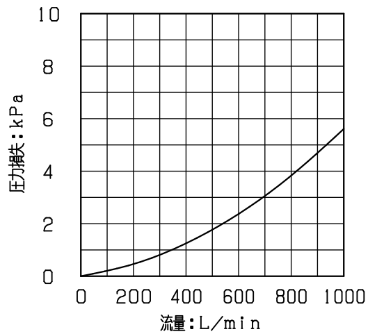
流量特性
