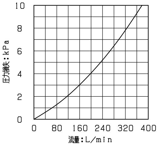
流量特性
