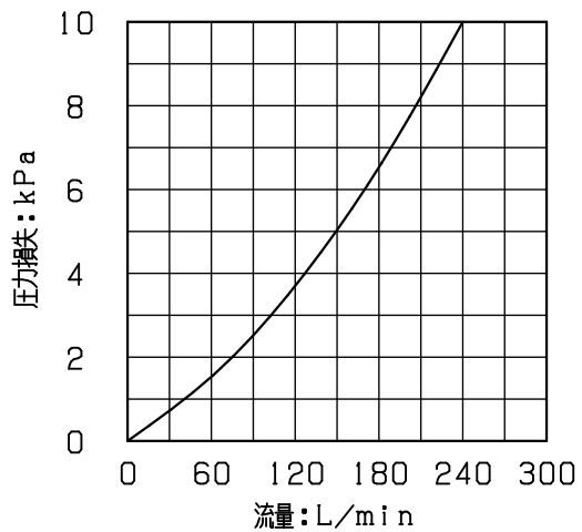
流量特性
