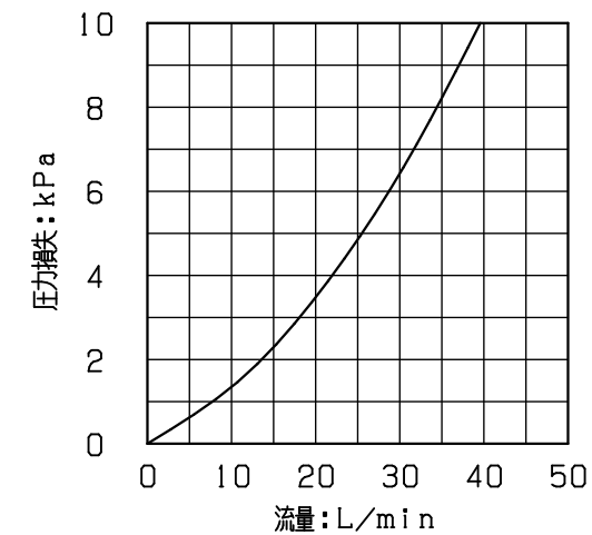
流量特性
