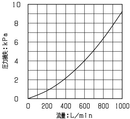
流量特性
