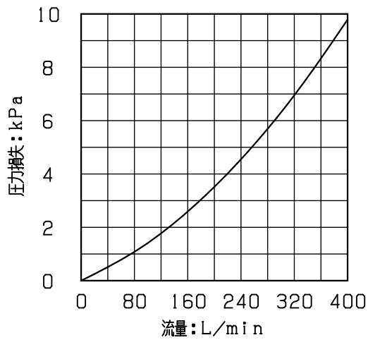
流量特性
