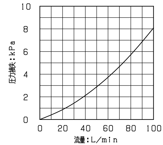
流量特性
